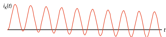
• Рис. 2. Осциллограмма тока КЗ, имеющего периодическую и аперриодическую составляющие
